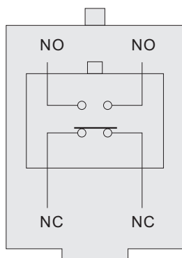
Konfiguracija kontakata
